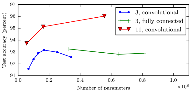
图 6.7: 参数数量的影响。更深的模型往往表现更好。这不仅仅是因为模型更大。Goodfellow et al. (2014d) 的这项实验表明，增加卷积网络层中参数的数量，但是不增加它们的深度，在提升测试集性能方面几乎没有效果，如此图所示。图例标明了用于画出每条曲线的网络深度，以及曲线表示的是卷积层还是全连接层的大小变化。我们可以观察到，在这种情况下，浅层模型在参数数量达到 2000 万时就过拟合，而深层模型在参数数量超过 6000 万时仍然表现良好。这表明，使用深层模型表达出了对模型可以学习的函数空间的有用偏好。具体来说，它表达了一种信念，即该函数应该由许多更简单的函数复合在一起而得到。这可能导致学习由更简单的表示所组成的表示（例如，由边所定义的角）或者学习具有顺序依赖步骤的程序（例如，首先定位一组对象，然后分割它们，之后识别它们）。
