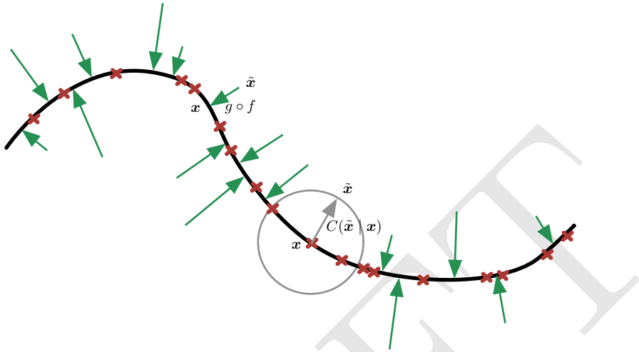
图 14.4: 去噪自编码器被训练为将损坏的数据点 \tilde{x} 映射回原始数据点 x 。我们将训练样本 x 表示为位于低维流形（粗黑线）附近的红叉。我们用灰色圆圈表示等概率的损坏过程 C(\tilde{x} | x) 。灰色箭头演示了如何将一个训练样本转换为经过此损坏过程的样本。当训练去噪自编码器最小化平方误差 \|g(f(\tilde{x})) - x\|^2 的平均值时，重构 g(f(\tilde{x})) 估计 \mathbb{E}_{x, \tilde{x} \sim p_{\text{data}}(x)C(\tilde{x}|x)}[x | \tilde{x}] 。 g(f(\tilde{x})) 对可能产生 \tilde{x} 的原始点 x 的质心进行估计，所以向量 g(f(\tilde{x})) - \tilde{x} 近似指向流形上最近的点。因此自编码器可以学习由绿色箭头表示的向量场 g(f(x)) - x 。该向量场将得分 \nabla_x \log p_{\text{data}}(x) 估计为一个乘性因子，即重构误差均方根的平均。
