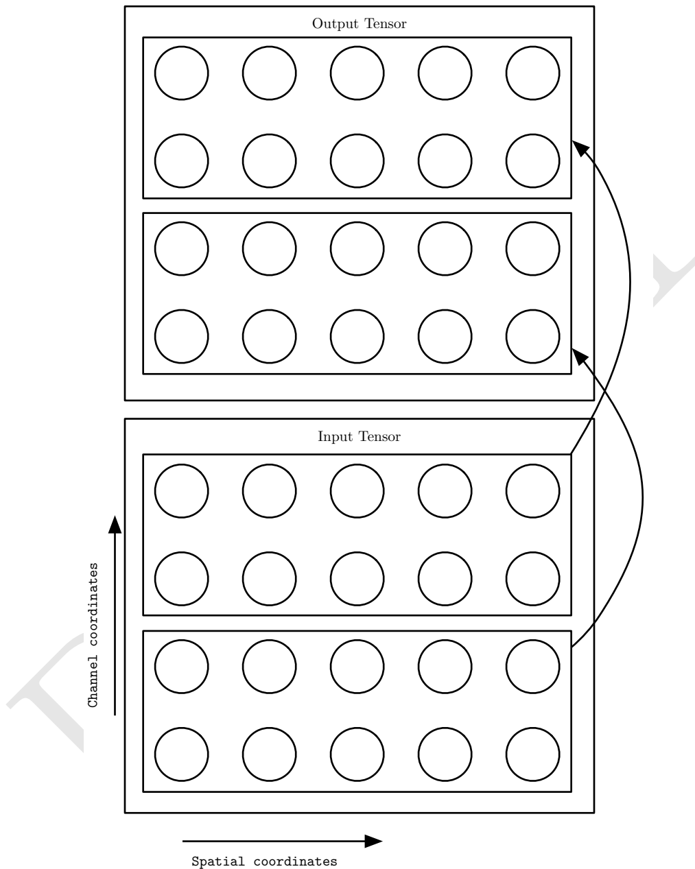
图 9.15: 卷积网络的前两个输出通道只和前两个输入通道相连，随后的两个输出通道只和随后的两个输入通道相连。
