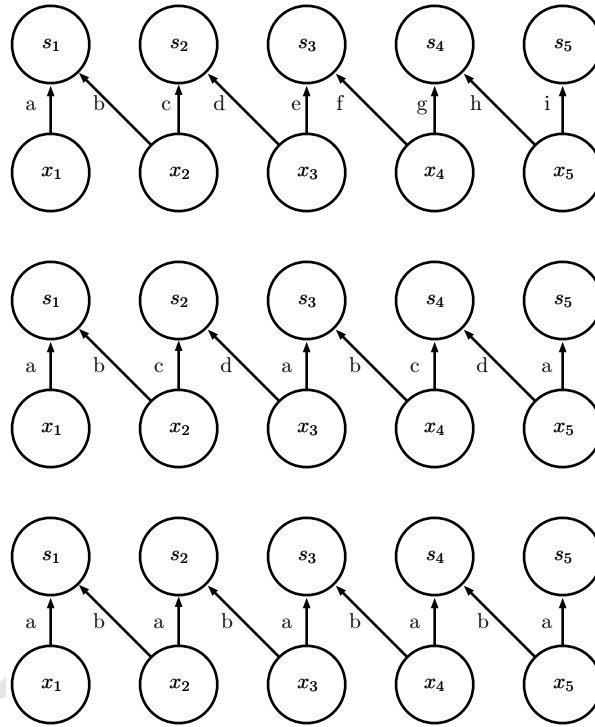
图 9.16: 局部连接层、平铺卷积和标准卷积的比较。当使用相同大小的核时，这三种方法在单元之间具有相同的连接。此图是对使用两个像素宽的核的说明。这三种方法之间的区别在于它们如何共享参数。(上) 局部连接层根本没有共享参数。我们对每个连接使用唯一的字母标记，来表明每个连接都有它自身的权重。(中) 平铺卷积有 t 个不同的核。这里我们说明 t = 2 的情况。其中一个核具有标记为“a”和“b”的边，而另一个具有标记为“c”和“d”的边。每当我们在输出中右移一个像素后，我们使用一个不同的核。这意味着，与局部连接层类似，输出中的相邻单元具有不同的参数。与局部连接层不同的是，在我们遍历所有可用的 t 个核之后，我们循环回到了第一个核。如果两个输出单元间隔 t 个步长的倍数，则它们共享参数。(下) 传统卷积等效于 t = 1 的平铺卷积。它只有一个核，并且被应用到各个地方，我们在图中表示为在各处使用具有标记为“a”和“b”的边的核。
