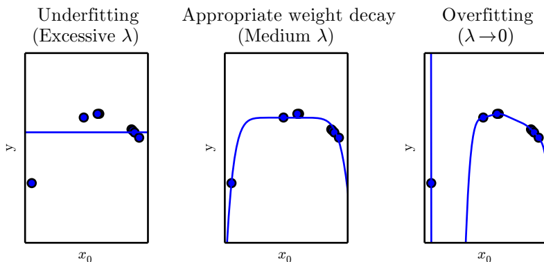
图 5.5: 我们使用高阶多项式回归模型来拟合图 5.2 中训练样本。真实函数是二次的，但是在这里我们只使用 9 阶多项式。我们通过改变权重衰减的量来避免高阶模型的过拟合问题。(左) 当 \lambda 非常大时，我们可以强迫模型学习到了一个没有斜率的函数。由于它只能表示一个常数函数，所以会导致欠拟合。(中) 取一个适当的 \lambda 时，学习算法能够用一个正常的形状来恢复曲率。即使模型能够用更复杂的形状来表示函数，权重衰减鼓励用一个带有更小参数的更简单的模型来描述它。(右) 当权重衰减趋近于 0 (即使用 Moore-Penrose 伪逆来解决这个带有最小正则化的欠定问题) 时，这个 9 阶多项式会导致严重的过拟合，这和我们图 5.2 中看到的一样。
