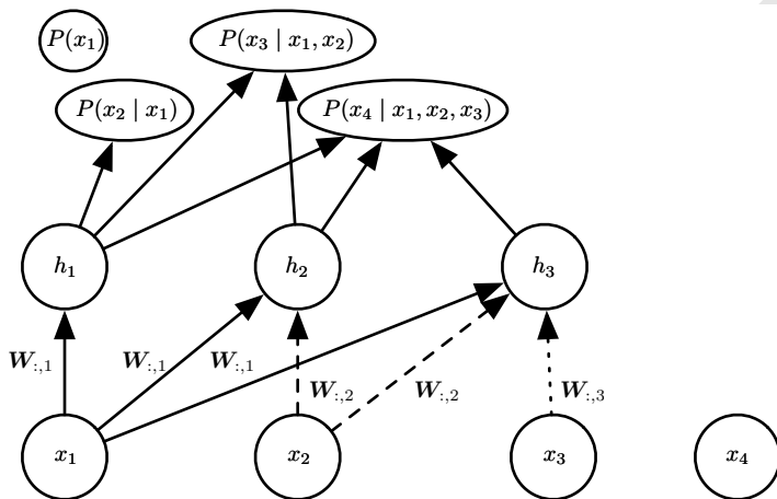
图 20.10: 神经自回归密度估计器 (NADE) 的示意图。隐藏单元被组织在组 h^{(j)} 中，使得只有输入 x_1, \dots, x_i 参与计算 h^{(i)} 和预测 P(x_j | x_{j-1}, \dots, x_1) (对于 j > i )。NADE 使用特定的权重共享模式区别于早期的神经自回归网络： W'_{j,k,i} = W_{k,i} 被共享于所有从 x_i 到任何 j \geq i 组中第 k 个单元的权重 (在图中使用相同的线型表示复制权重的每个实例)。注意向量 (W_{1,i}, W_{2,i}, \dots, W_{n,i}) 记为 W_{:,i} 。
