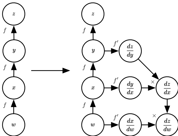
图 6.10: 使用符号到符号的方法计算导数的示例。在这种方法中，反向传播算法不需要访问任何实际的特定数值。相反，它将节点添加到计算图中来描述如何计算这些导数。通用图形求值引擎可以在随后计算任何特定数值的导数。(左) 在这个例子中，我们从表示 z = f(f(f(w))) 的图开始。(右) 我们运行反向传播算法，指导它构造表达式 \frac{dz}{dw} 对应的图。在这个例子中，我们不解释反向传播算法如何工作。我们的目的只是说明想要的结果是什么：符号描述的导数的计算图。
