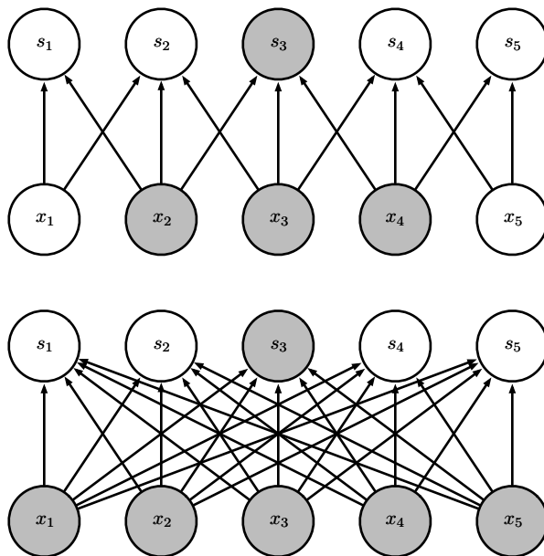
图 9.3: 稀疏连接, 对每幅图从上往下看。我们强调了一个输出单元 s_3 以及 x 中影响该单元的输入单元。这些单元被称为 s_3 的接受域 (receptive field) 3 。(上) 当 s 是由核宽度为 3 的卷积产生时, 只有三个输入影响 s_3 。(下) 当 s 是由矩阵乘法产生时, 连接不再是稀疏的, 所以所有的输入都会影响 s_3 。
