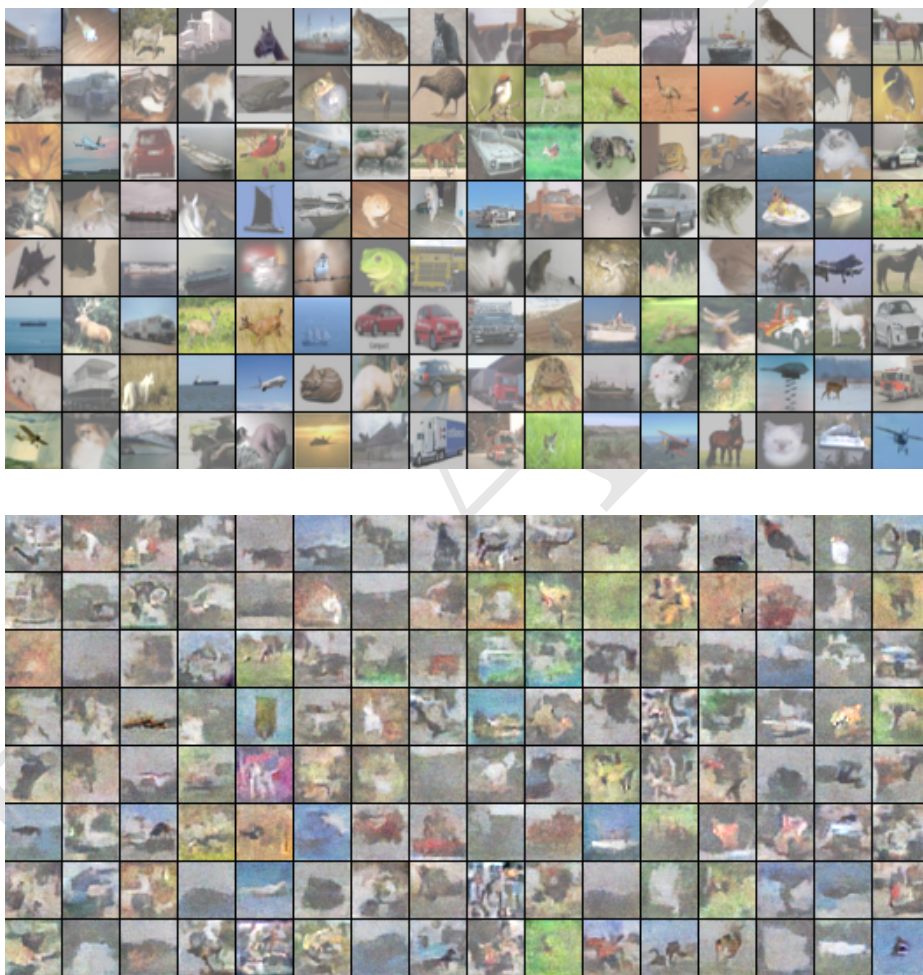
图 16.1: 自然图片的概率建模。(上) CIFAR-10 数据集 (Krizhevsky and Hinton, 2009) 中的 32 \times 32 像素的样例图片。(下) 从这个数据集上训练的结构化概率模型中抽出的样本。每一个样本都出现在与其欧式距离最近的训练样本的格点中。这种比较使得我们发现这个模型确实能够生成新的图片，而不是记住训练样本。为了方便展示，两个集合的图片都经过了微调。图片经 Courville et al. (2011a) 许可转载。
