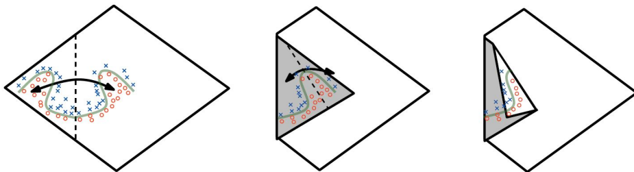
图 6.5: 关于更深的整流网络具有指数优势的一个直观的几何解释，来自 Montufar et al. (2014)。(左)绝对值整流单元对其输入中的每对镜像点有相同的输出。镜像的对称轴由单元的权重和偏置定义的超平面给出。在该单元顶部计算的函数（绿色决策面）将是横跨该对称轴的更简单模式的一个镜像。(中) 该函数可以通过折叠对称轴周围的空间来得到。(右) 另一个重复模式可以在第一个的顶部折叠（由另一个下游单元）以获得另外的对称性（现在重复四次，使用了两个隐藏层）。经 Montufar et al. (2014) 许可改编此图。
