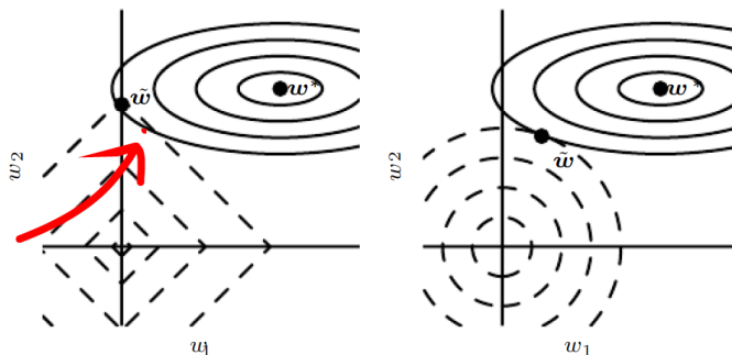
图 7.4: 提前终止效果的示意图。(左) 实线轮廓线表示负对数似然的轮廓。虚线表示从原点开始的 SGD 所经过的轨迹。提前终止的轨迹在较早的点 \tilde{\mathbf{w}} 处停止，而不是停止在最小化代价的点 \mathbf{w}^* 处。(右) 为了对比，使用 L^2 正则化效果的示意图。虚线圆圈表示 L^2 惩罚的轮廓， L^2 惩罚使得总代价的最小值比非正则化代价的最小值更靠近原点。
