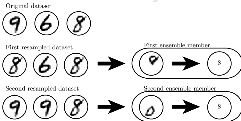
图 7.5: 描述Bagging如何工作的草图。假设我们在上述数据集（包含一个 8, 一个 6 和一个 9）上训练数字 8 的检测器。假设我们制作了两个不同的重采样数据集。Bagging训练程序通过替换采样构建这些数据集。第一个数据集忽略 9 并重复 8。在这个数据集上，检测器得知数字顶部有一个环就对应于一个 8。第二个数据集中，我们忽略 6 并重复 9。在这种情况下，检测器得知数字底部有一个环就对应于一个 8。这些单独的分类规则中的每一个都是不可靠的，但如果我们平均它们的输出，就能得到鲁棒的检测器，只有当 8 的两个环都存在时才能实现最大置信度。
