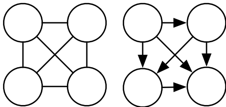
图 16.10: 完全图的例子，完全图能够描述任何的概率分布。这里我们展示了一个带有四个随机变量的例子。(左) 完全无向图。在无向图中，完全图是唯一的。(右) 一个完全有向图。在有向图中，并不存在唯一的完全图。我们选择一种变量的排序，然后对每一个变量，从它本身开始，向每一个指向顺序在其后面的变量画一条弧。因此存在着关于变量数阶乘数量级的不同种完全图。在这个例子中，我们是从左到右从上到下地排序变量。
