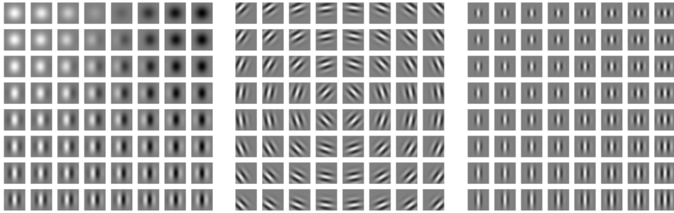
图 9.18: 具有各种参数设置的Gabor 函数。白色表示大的正权重，黑色表示大的负权重，背景灰色对应于零权重。(左) 控制坐标系的参数具有不同值的Gabor 函数，这些参数包括： x_0 、 y_0 和 \gamma 。在该网格中的每个Gabor 函数被赋予和它在网格中的位置成比例的 x_0 和 y_0 的值，并且 \tau 被选择为使得每个 Gabor 过滤器对从网格中心辐射出的方向非常敏感。对于其他两幅图， x_0 、 y_0 和 \gamma 固定为零。(中) 具有不同高斯比例参数 \beta_x 和 \beta_y 的Gabor 函数。当我们从左到右通过网格时，Gabor 函数被设置为增加宽度（减少 \beta_x ）；当我们从上到下通过网格时，Gabor 函数被设置为增加高度（减少 \beta_y ）。对于其他两幅图， \beta 值固定为图像宽度的 1.5 倍。(右) 具有不同的正弦参数 f 和 \phi 的Gabor 函数。当我们从上到下移动时， f 增加；当我们从左到右移动时， \phi 增加。对于其他两幅图， \phi 固定为 0， f 固定为图像宽度的 5 倍。
