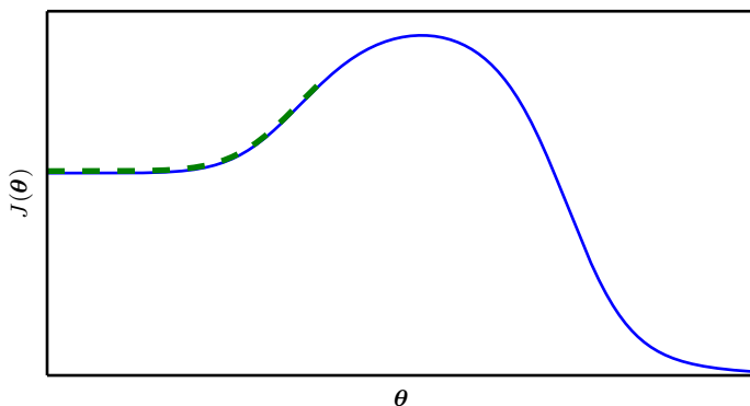
图 8.4: 如果局部表面没有指向全局解，基于局部下坡移动的优化可能会失败。这里我们提供一个例子，说明即使在没有鞍点或局部极小值的情况下，优化过程会如何失败。此例中的代价函数仅包含朝向低值而不是极小值的渐近线。在这种情况下，造成这种困难的主要原因是初始化在“山”的错误一侧，并且无法遍历。在高维空间中，学习算法通常可以环绕过这样的高山，但是相关的轨迹可能会很长，并且导致过长的训练时间，如图 8.2 所示。
