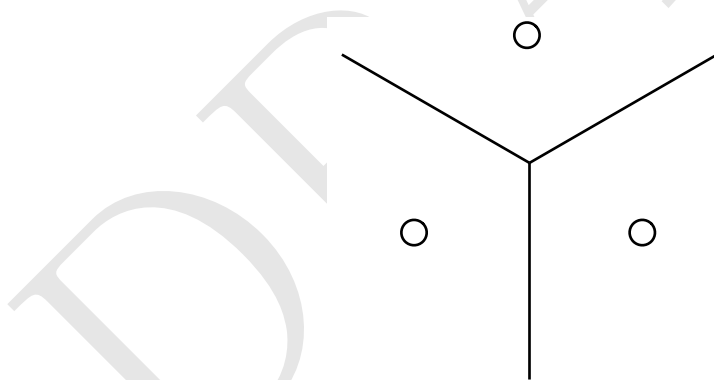
图 5.10: 最近邻算法如何划分输入空间的示例。每个区域内的一个样本（这里用圆圈表示）定义了区域边界（这里用线表示）。每个样本相关的 y 值定义了对应区域内所有数据点的输出。由最近邻定义并且匹配几何模式的区域被称为 Voronoi 图。这些连续区域的数量不会比训练样本的数量增加得更快。尽管此图具体说明了最近邻算法的效果，其他的单纯依赖局部光滑先验的机器学习算法也表现出了类似的泛化能力：每个训练样本仅仅能告诉学习者如何在其周围的相邻区域泛化。
