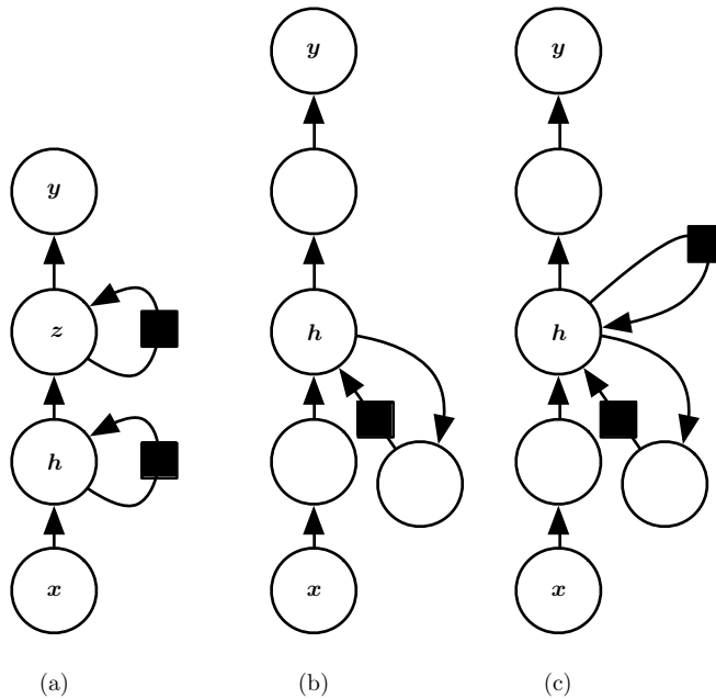
图 10.13: 循环神经网络可以通过许多方式变得更深 (Pascanu et al. , 2014a)。(a) 隐藏循环状态可以被分解为具有层次的组。(b) 可以向输入到隐藏，隐藏到隐藏以及隐藏到输出的部分引入更深的计算 (如 MLP)。这可以延长链接不同时间步的最短路径。(c) 可以引入跳跃连接来缓解路径延长的效应。
