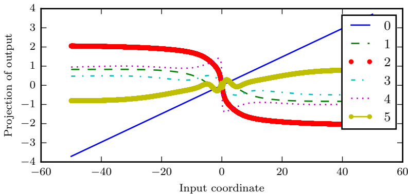
图 10.15: 重复组合函数。当组合许多非线性函数（如这里所示的线性 tanh 层）时，结果是高度非线性的，通常大多数值与微小的导数相关联，也有一些具有大导数的值，以及在增加和减小之间的多次交替。此处，我们绘制从 100 维隐藏状态降到单个维度的线性投影，绘制于 y 轴上。 x 轴是 100 维空间中沿着随机方向的初始状态的坐标。因此，我们可以将该图视为高维函数的线性截面。曲线显示每个时间步之后的函数，或者等价地，转换函数被组合一定次数之后。
