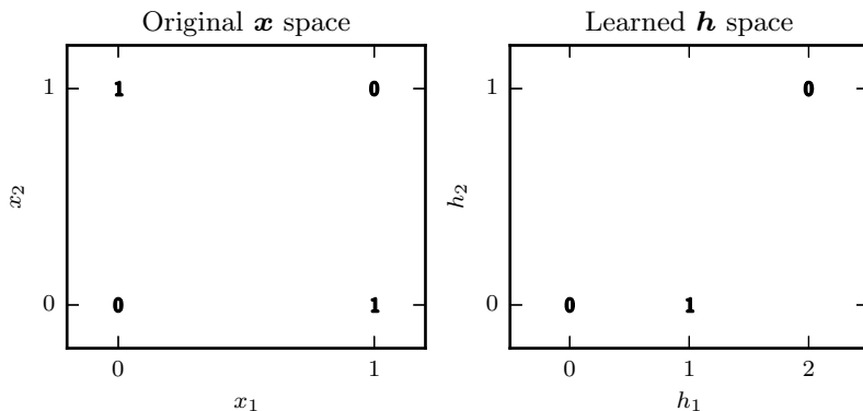
图 6.1: 通过学习一个表示来解决 XOR 问题。图上的粗体数字标明了学得的功能必须在每个点输出的值。(左) 直接应用于原始输入的线性模型不能实现 XOR 函数。当 x_1 = 0 时, 模型的输出必须随着 x_2 的增大而增大。当 x_1 = 1 时, 模型的输出必须随着 x_2 的增大而减小。线性模型必须对 x_2 使用固定的系数 w_2 。因此, 线性模型不能使用 x_1 的值来改变 x_2 的系数, 从而不能解决这个问题。(右) 在由神经网络提取的特征表示的变换空间中, 线性模型现在可以解决这个问题了。在我们的示例解决方案中, 输出必须为 1 的两个点折叠到了特征空间中的单个点。换句话说, 非线性特征将 \mathbf{x} = [1, 0]^T 和 \mathbf{x} = [0, 1]^T 都映射到了特征空间中的单个点 \mathbf{h} = [1, 0]^T 。线性模型现在可以将函数描述为 h_1 增大和 h_2 减小。在该示例中, 学习特征空间的动机仅仅是使得模型的能力更大, 使得它可以拟合训练集。在更现实的应用中, 学习的表示也可以帮助模型泛化。
