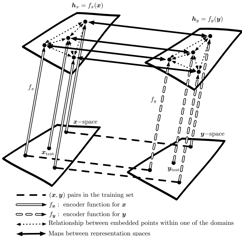
图 15.3: 两个域 x 和 y 之间的迁移学习能够进行零次学习。标注或未标注样本 x 可以学习表示函数 f_x 。同样地，样本 y 也可以学习表示函数 f_y 。上图中 f_x 和 f_y 旁都有一个向上的箭头，不同的箭头表示不同的作用函数。并且箭头的类型表示使用了哪一种函数。 h_x 空间中的相似性度量表示 x 空间中任意点对之间的距离，这种度量方式比直接度量 x 空间的距离更好。同样地， h_y 空间中的相似性度量表示 y 空间中任意点对之间的距离。这两种相似函数都使用带点的双向箭头表示。标注样本（水平虚线） (x, y) 能够学习表示 f_x(x) 和表示 f_y(y) 之间的单向或双向映射（实双向箭头），以及这些表示之间如何锚定。零数据学习可以通过以下方法实现。像 x_{\text{test}} 可以和单词 y_{\text{test}} 关联起来，即使该单词没有像，仅仅是因为单词表示 f_y(y_{\text{test}}) 和像表示 f_x(x_{\text{test}}) 可以通过表示空间的映射彼此关联。这种方法有效的原因是，尽管像和单词没有匹配成对，但是它们各自的特征向量 f_x(x_{\text{test}}) 和 f_y(y_{\text{test}}) 互相关联。上图受 Hrant Khachatrian 的建议启发。
