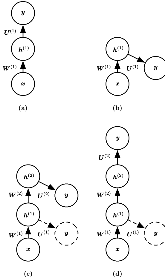
图 8.7: 一种形式的贪心监督预训练的示意图 (Bengio et al. , 2007a)。 (a) 我们从训练一个足够浅的架构开始。 (b) 同一个架构的另一描绘。 (c) 我们只保留原始网络的输入到隐藏层, 并丢弃隐藏到输出层。我们将第一层隐藏层的输出作为输入发送到另一监督单隐层 MLP (使用与第一个网络相同的目标训练), 从而可以添加第二层隐藏层。这可以根据需要重复多层。 (d) 所得架构的另一种描绘, 可视为前馈网络。为了进一步改进优化, 我们可以联合地精调所有层 (仅在该过程的结束或者该过程的每个阶段)。
