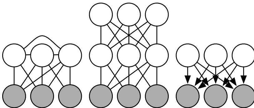
图 19.1: 深度学习中难以处理的推断问题通常是由于结构化图模型中潜变量的相互作用。这些相互作用产生于一个潜变量与另一个潜变量或者当V-结构的子节点可观察时与更长的激活路径相连。(左) 一个隐藏单元存在连接的半受限玻尔兹曼机 (semi-restricted Boltzmann Machine) (Osindero and Hinton, 2008)。由于存在大量潜变量的团, 潜变量的直接连接使得后验分布难以处理。(中) 一个深度玻尔兹曼机, 被分层从而使得不存在层内连接, 由于层之间的连接其后验分布仍然难以处理。(右) 当可见变量可观察时这个有向模型的潜变量之间存在相互作用, 因为每两个潜变量都是共父。即使拥有上图中的某一种结构, 一些概率模型依然能够获得易于处理的关于潜变量的后验分布。如果我们选择条件概率分布来引入相对于图结构描述的额外的独立性这种情况也是可能出现的。举个例子, 概率 PCA 的图结构如右图所示, 然而由于其条件分布的特殊性质 (带有相互正交基向量的线性高斯条件分布) 依然能够进行简单的推断。
