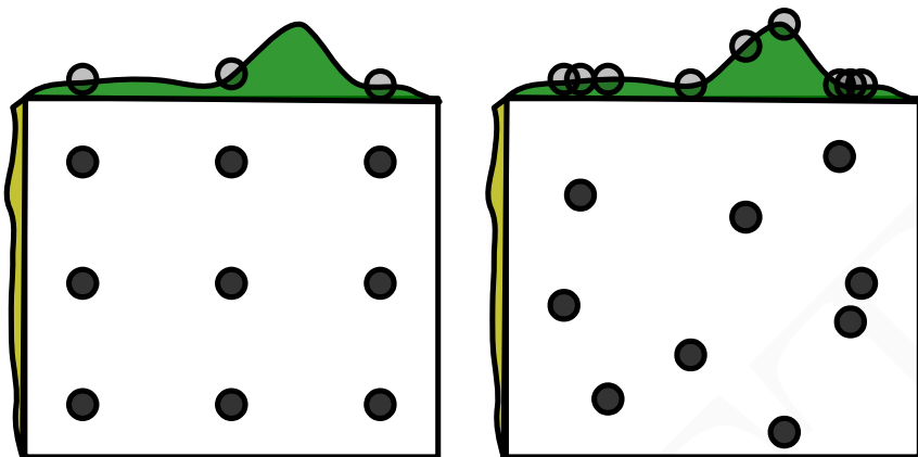
图 11.2: 网格搜索和随机搜索的比较。为了方便地说明, 我们只展示两个超参数的例子, 但是我们关注的问题中超参数个数通常会更多。(左) 为了实现网格搜索, 我们为每个超参数提供了一个值的集合。搜索算法对每一种在这些集合的交叉积中的超参数组合进行训练。(右) 为了实现随机搜索, 我们给联合超参数赋予了一个概率分布。通常超参数之间是相互独立的。常见的这种分布的选择是均匀分布或者是对数均匀(从对数均匀分布中抽样, 就是对从均匀分布中抽取的样本进行指数运算)的。然后这些搜索算法从联合的超参数空间中采样, 然后运行每一个样本。网格搜索和随机搜索都运行了验证集上的误差并返回了最优的解。这个图说明了通常只有一个超参数对结果有着重要的影响。在这个例子中, 只有水平轴上的超参数对结果有重要的作用。网格搜索将大量的计算浪费在了指数量级的对结果无影响的超参数中, 相比之下随机搜索几乎每次测试都测试了对结果有影响的每个超参数的独一无二的值。此图经 Bergstra and Bengio (2011) 允许转载。
