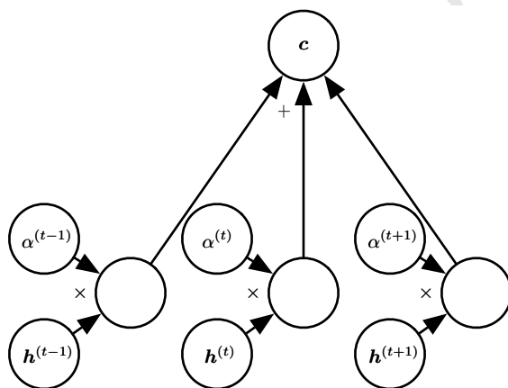
图 12.6: 由 Bahdanau et al. (2015) 引入的现代注意力机制，本质上是加权平均。注意力机制对具有权重 \alpha^{(t)} 的特征向量 h^{(t)} 进行加权平均形成上下文向量 c 。在一些应用中，特征向量 h 是神经网络的隐藏单元，但它们也可以是模型的原始输入。权重 \alpha^{(t)} 由模型本身产生。它们通常是区间 [0, 1] 中的值，并且旨在仅仅集中在单个 h^{(t)} 周围，使得加权平均精确地读取接近一个特定时间步的特征向量。权重 \alpha^{(t)} 通常由模型另一部分发出的相关性得分应用 softmax 函数后产生。注意力机制在计算上需要比直接索引期望的 h^{(t)} 付出更高的代价，但直接索引不能使用梯度下降训练。基于加权平均的注意力机制是平滑、可微的近似，可以使用现有优化算法训练。
